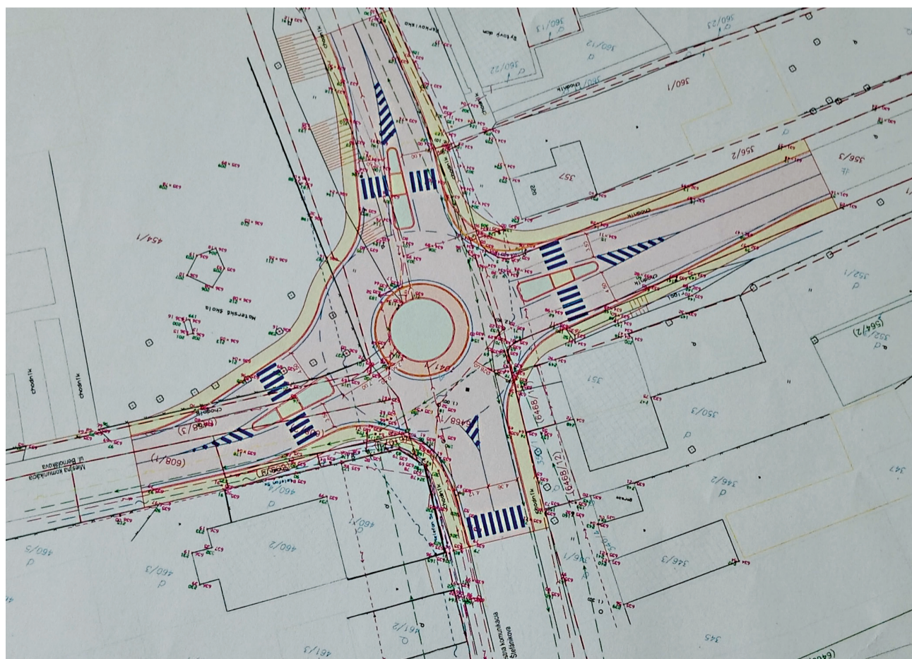
Projekt riešenia novej kruhovej križovatky na Štefánikovej ulici, nad Lidlom, vedľa MŠ.
